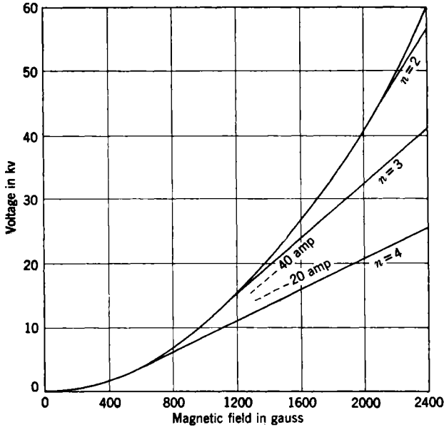
FIG. 1-26.—Hartree diagram.
